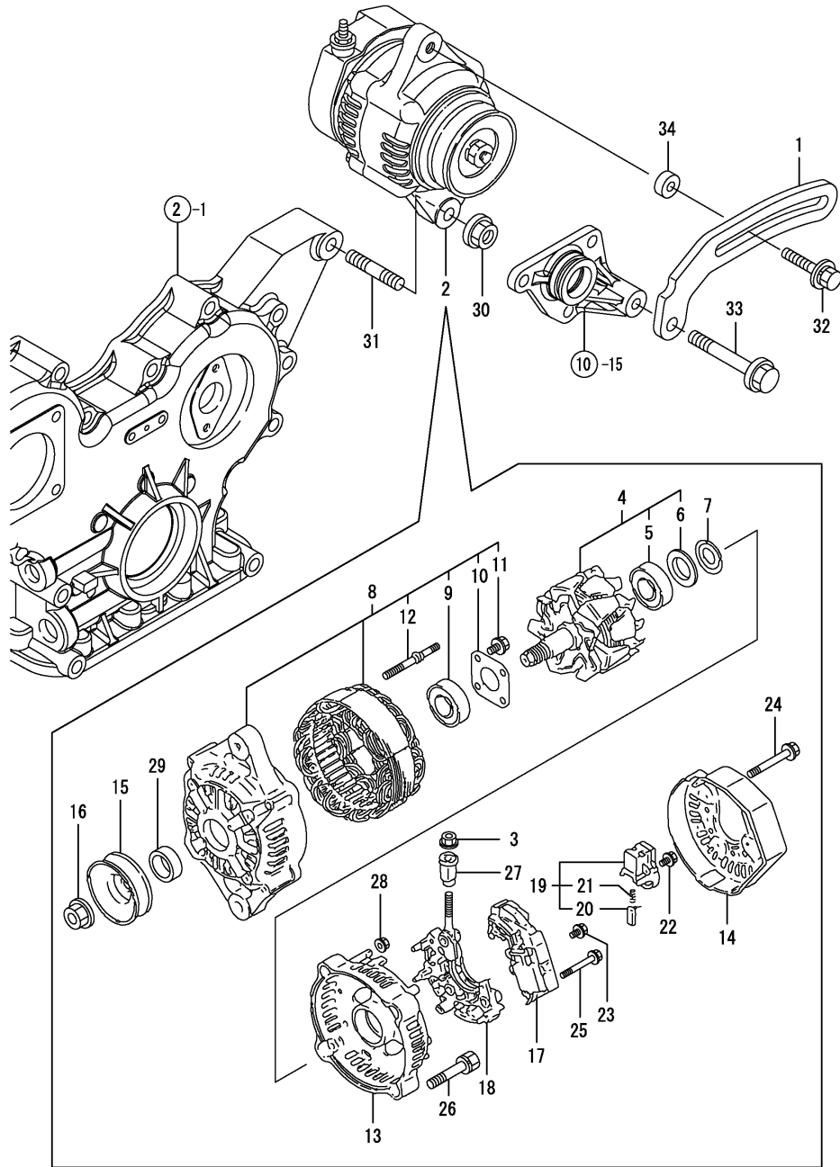
Fig.16. GENERATOR
