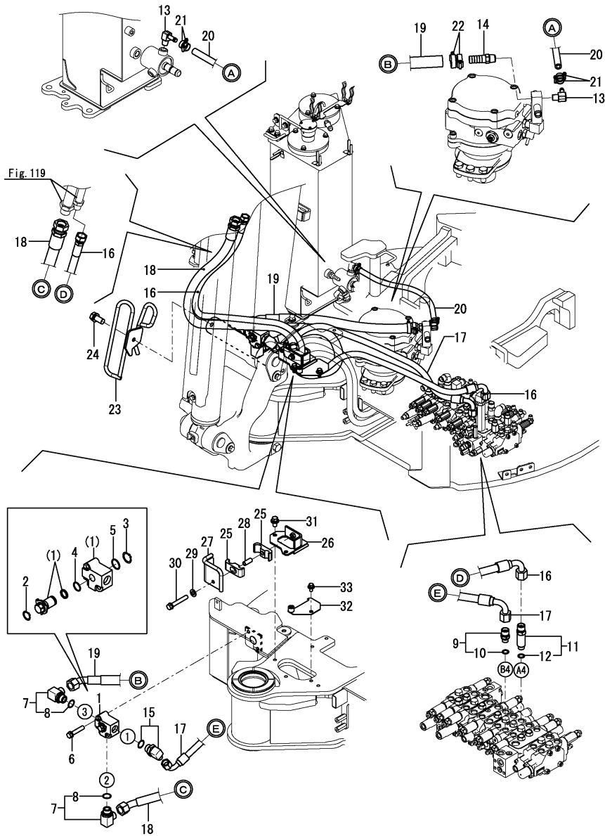
Fig.118. P.T.O.(CONTROL VALVE - BOOM)
