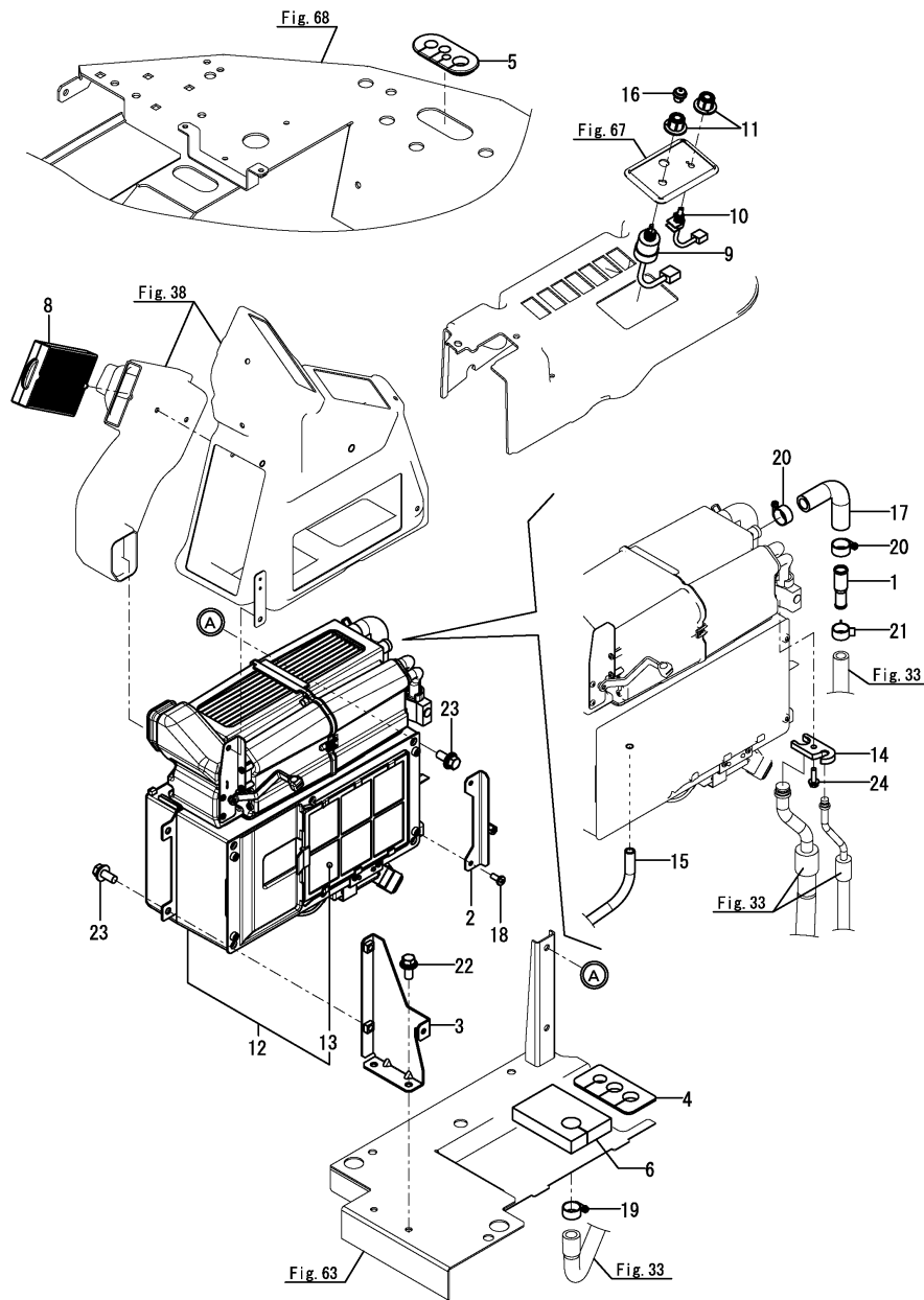
Fig.32. AIR CONDITIONER(UNIT)
