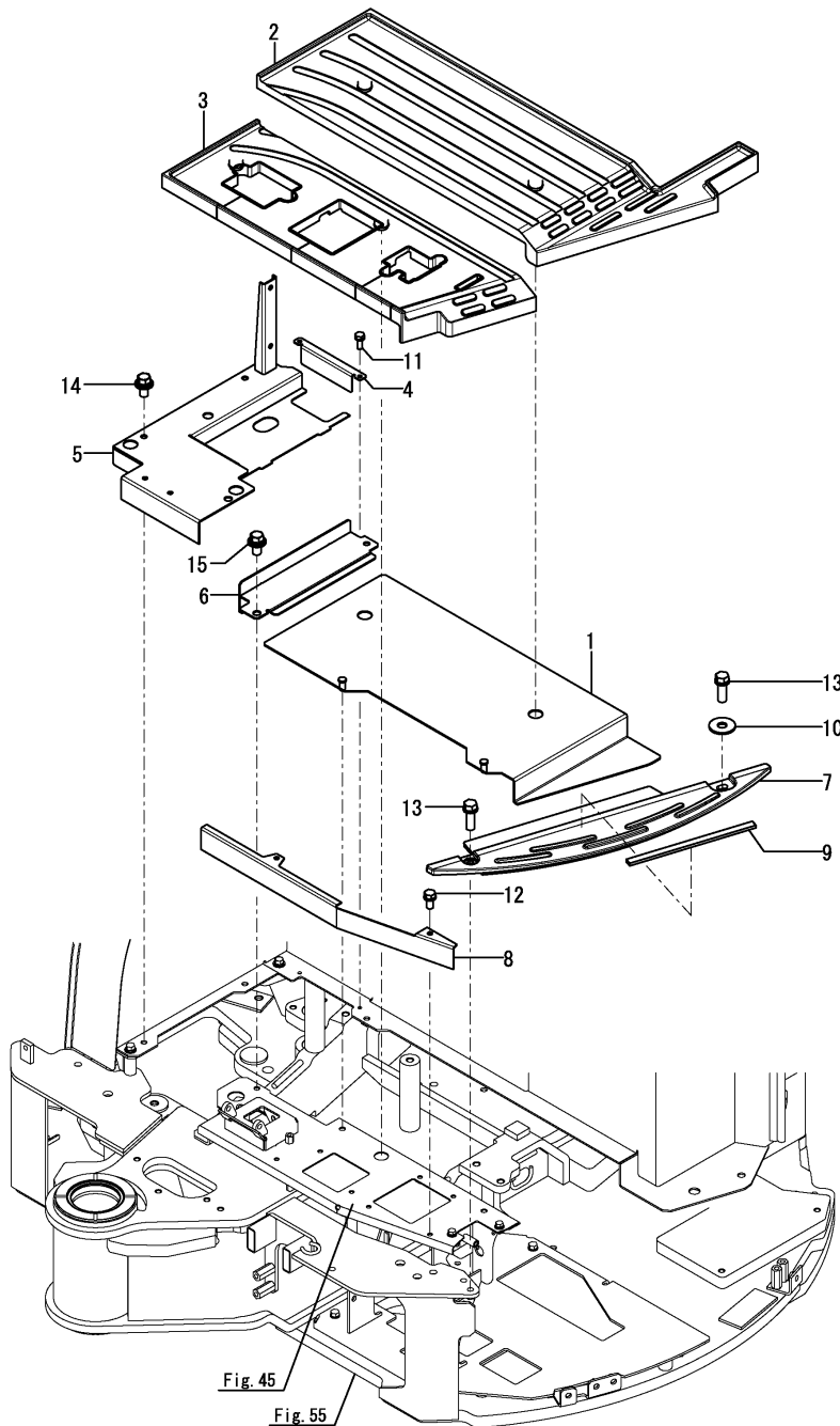
Fig.63. STEP(CABIN)
