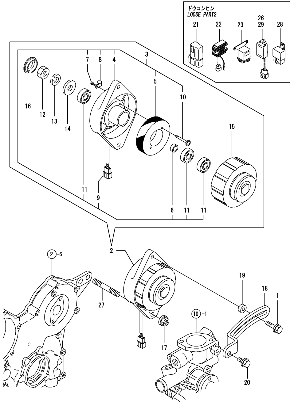
Fig.16. GENERATOR
